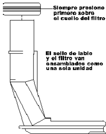
Filtro con sello de labio
